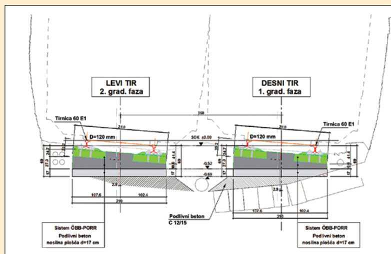
Karakteristični profil - Predor Križiški (vir Tiring, SŽ - ŽGP Ljubljana d.d.)
